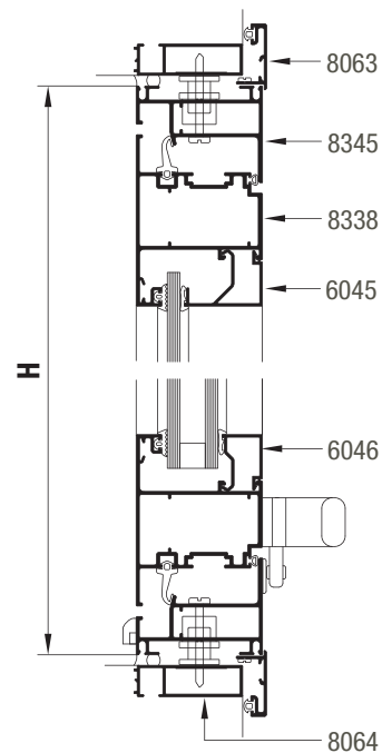
SECCION 3-4
