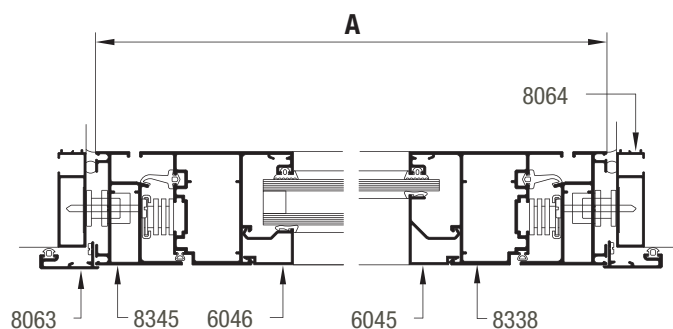
SECCION 1-2
