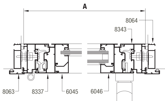
SECCION 1-2
