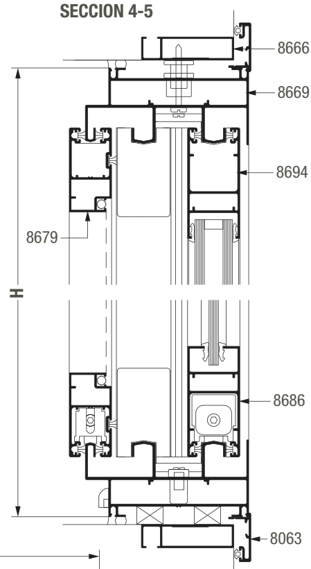
SECCION 4-5
