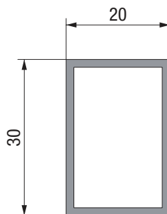
MC-145 0,381 Kg/m
