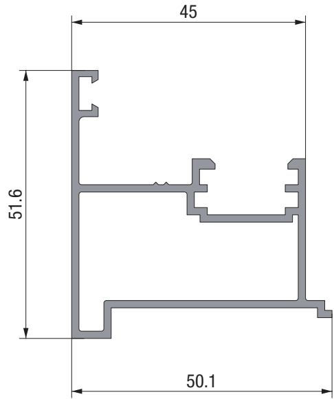
6224 0,794 Kg/m
