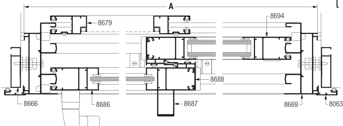
SECCIÓN 1-6-3
