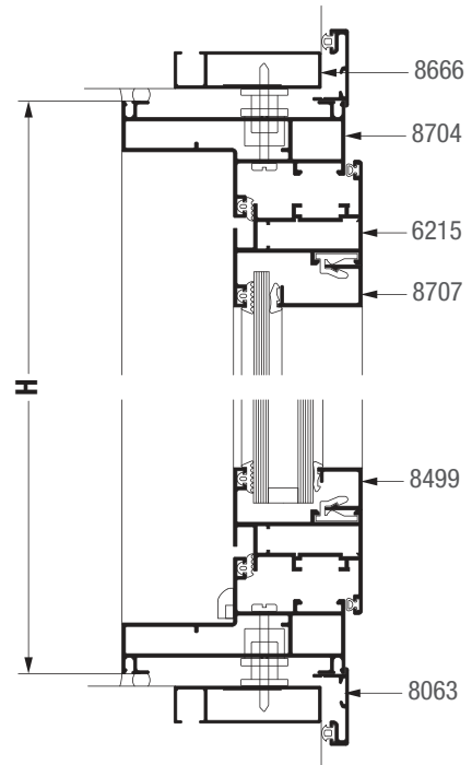
SECCION 3-4
